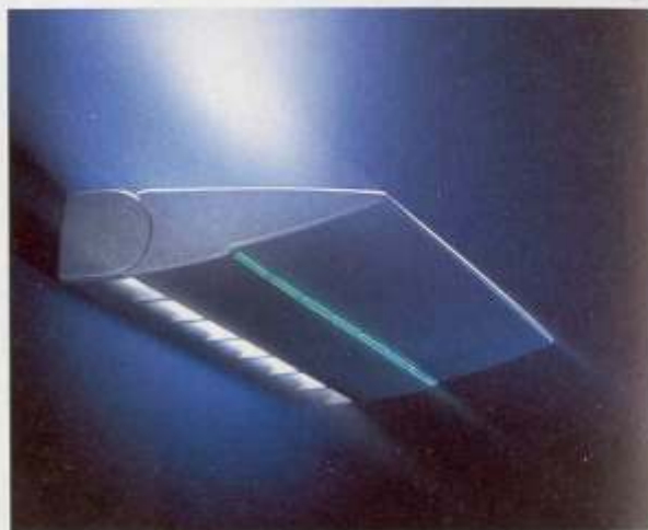
Als Wandleuchte (62,5x31,2 cm) erhält "Arianne" 2x36-W-Röhren. Auch hier strahlt das "Hauptlicht" nach oben, so daß indirektes Licht entsteht.
